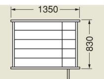
NM-45 (4.5尺) 天然銘木櫨 (小扉左・右兼用) W1350×H830×D440mm 119,000円
