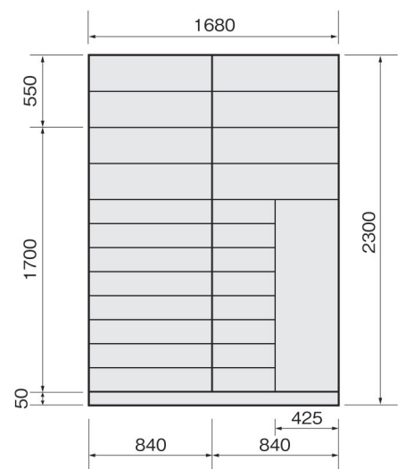
玄関収納 MA-1680・SU-1680 内部図
