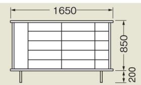
葵 1650 クリアー (タモ玉杵 タモ突き板 扉の戸枠無垢) W1650×H850×D430mm 298,000円
