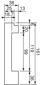
側面図
